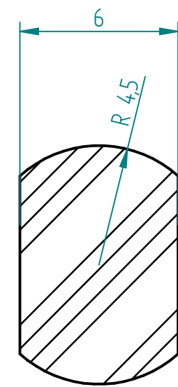
CORTE C-C
