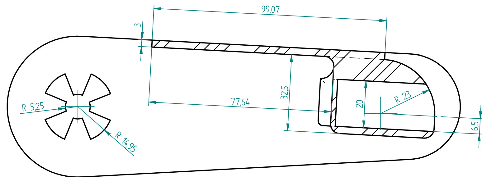
CORTE F-F
