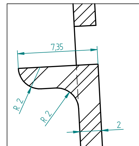
CORTE O-O Escala 5:1
