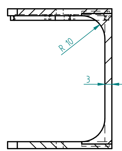
CORTE R-R
