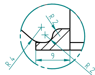
DETALLE T Escala 2:1
