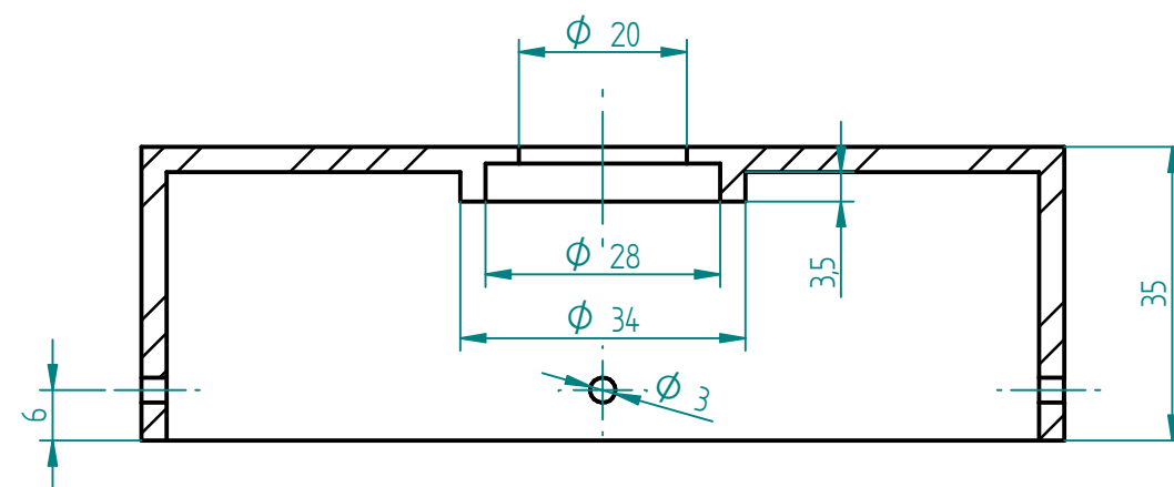
CORTE E-E
