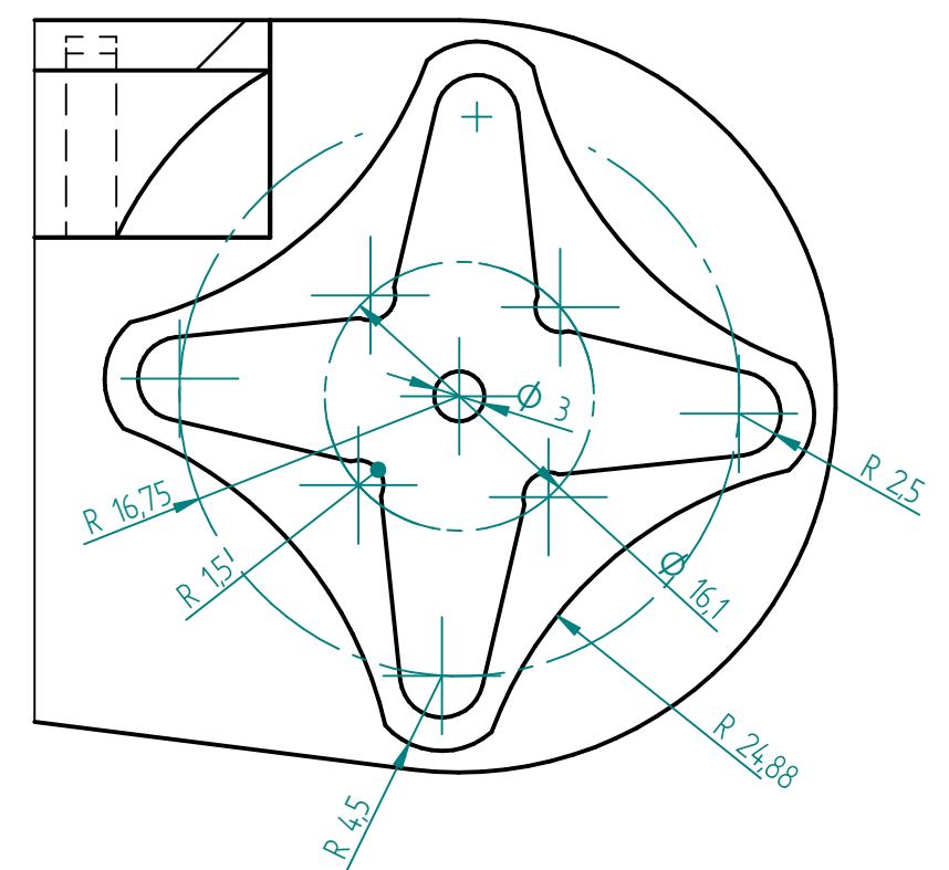
CORTE P-P Escala 2:1
